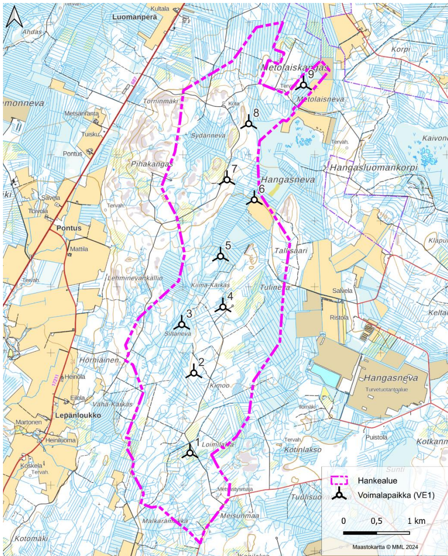
Kuva 1. Siltanevan tuulivoimahankkeen voimaloiden sijainnit hankevaihtoehtoon VE1 tilanteessa.
