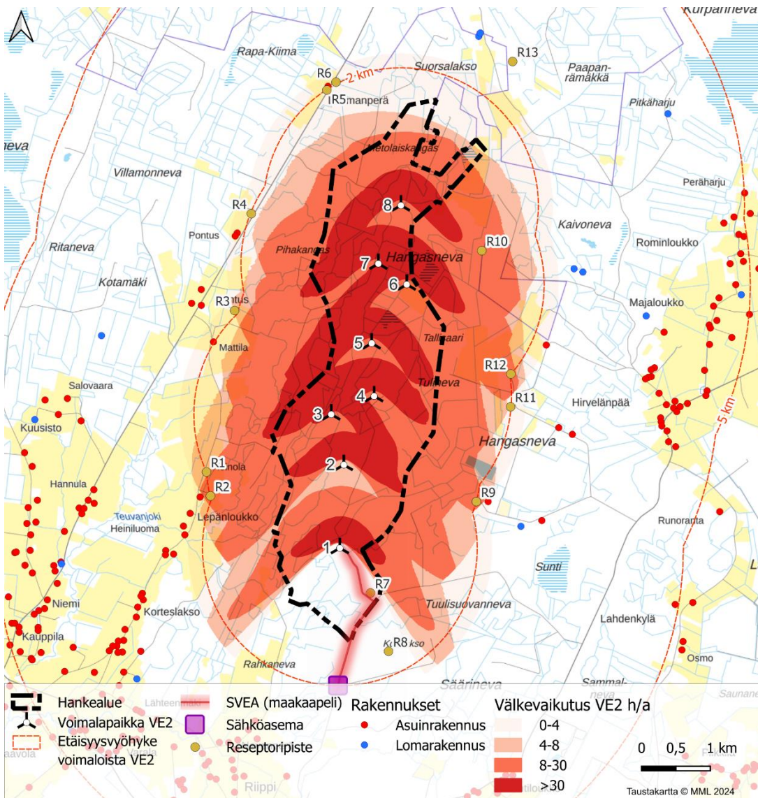
Kuva 5. Siltanevan hankevaihtoehdon VE2 mallinnustulosten mukainen välkevyöhykekartta ns. todellisen tilanteen vuotuiselle välkeajalle. Mallinnus tehty ilman puuston suojaavan vaikutuksen huomioimista.
